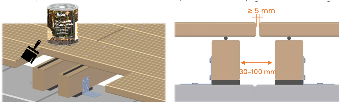
Figur 5: Terrassebræt, forsejlet med Kebony-endorseglingsvoks og monteret med Kebony-afstandsband, samlet over to bjælker. Denne metode sikrer en lang levetid og forenkler rengøringen.
