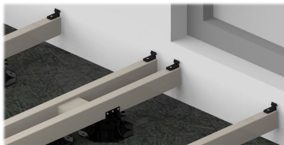
Figur 15: Monter pladen på underkonstruktionen, og tryk clipsen ind i holderne.
